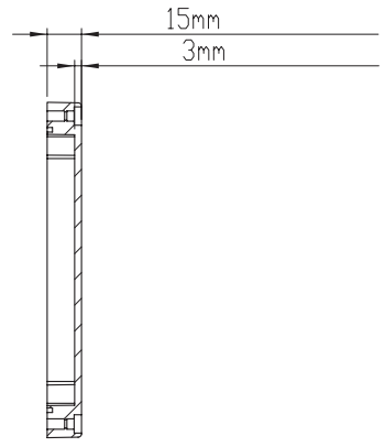
SECTION B-B SCALE 2 : 5
